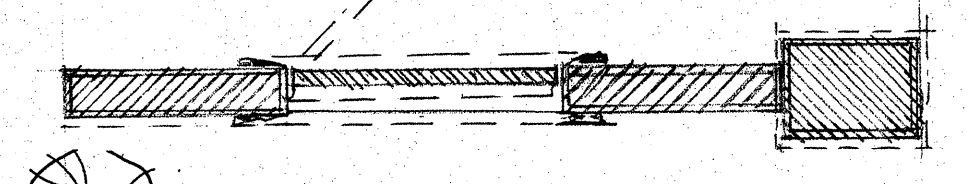
H. S. R. DOOR SCALE 1/2" = 1'-0"
