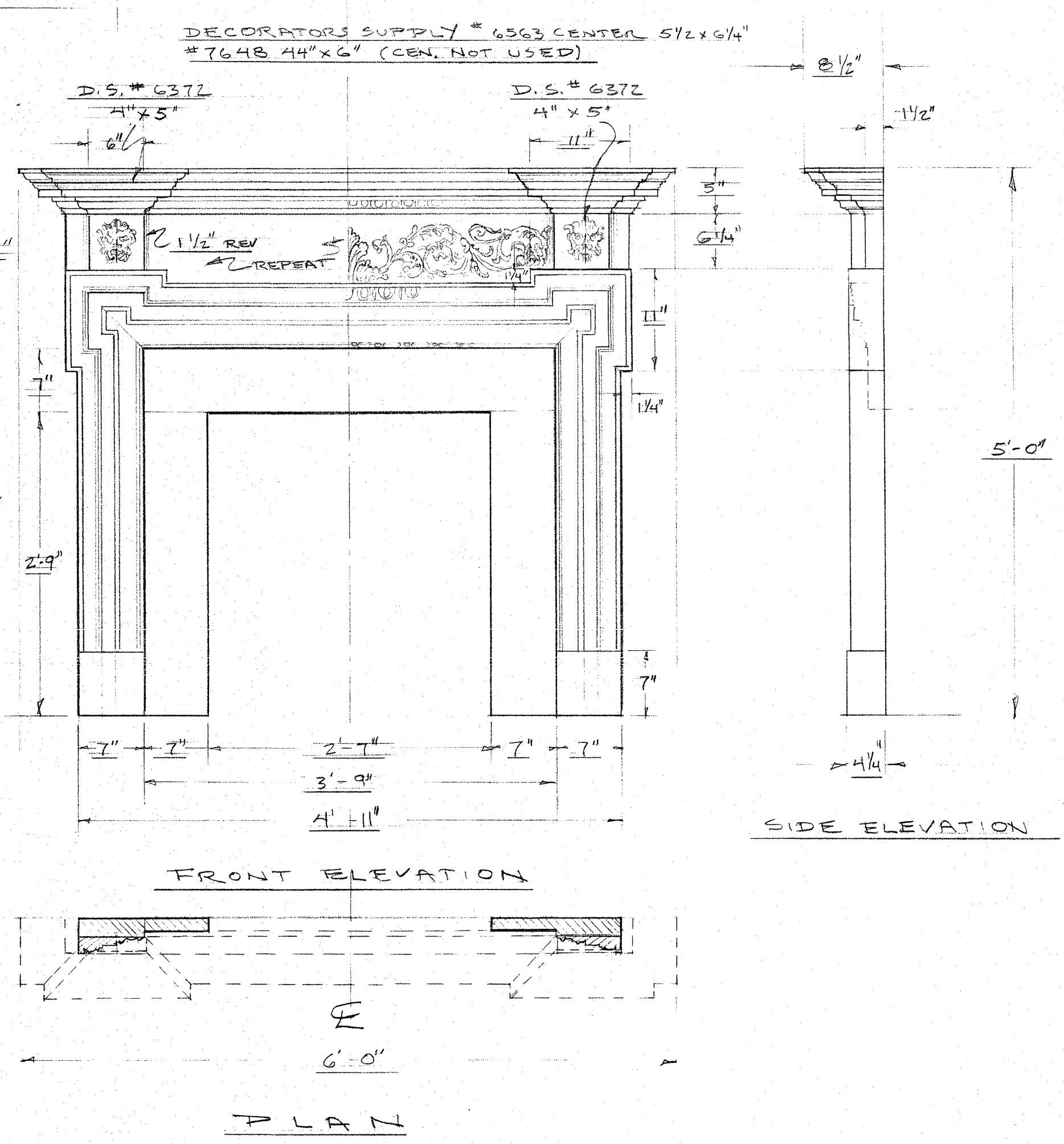
D1 FIREPLACE + MANTEL SCALE: 1" = 1'-0" DETAIL # 1
