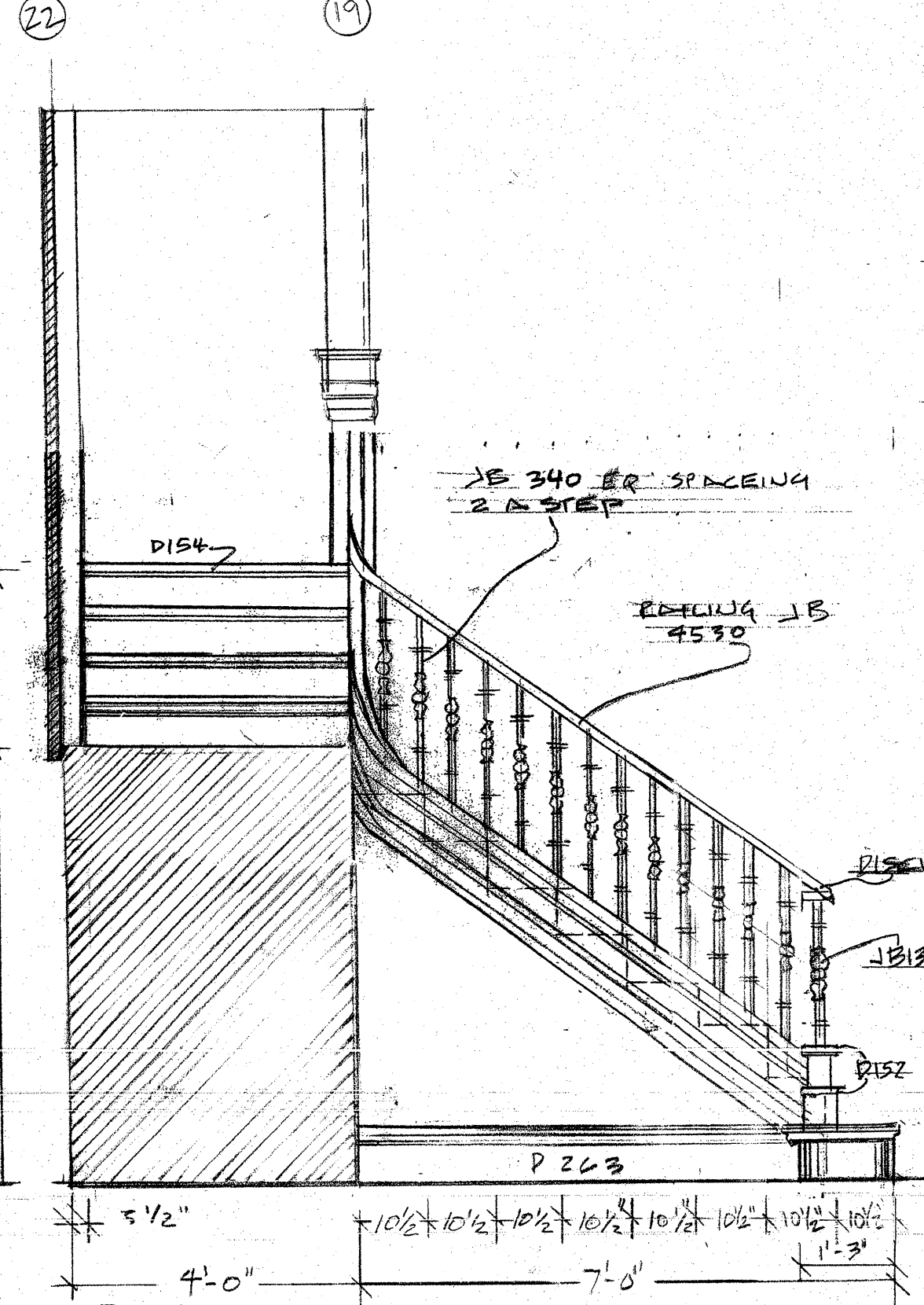
AA. STAIR SECTION SCALE 1/2" = 1'-0"
