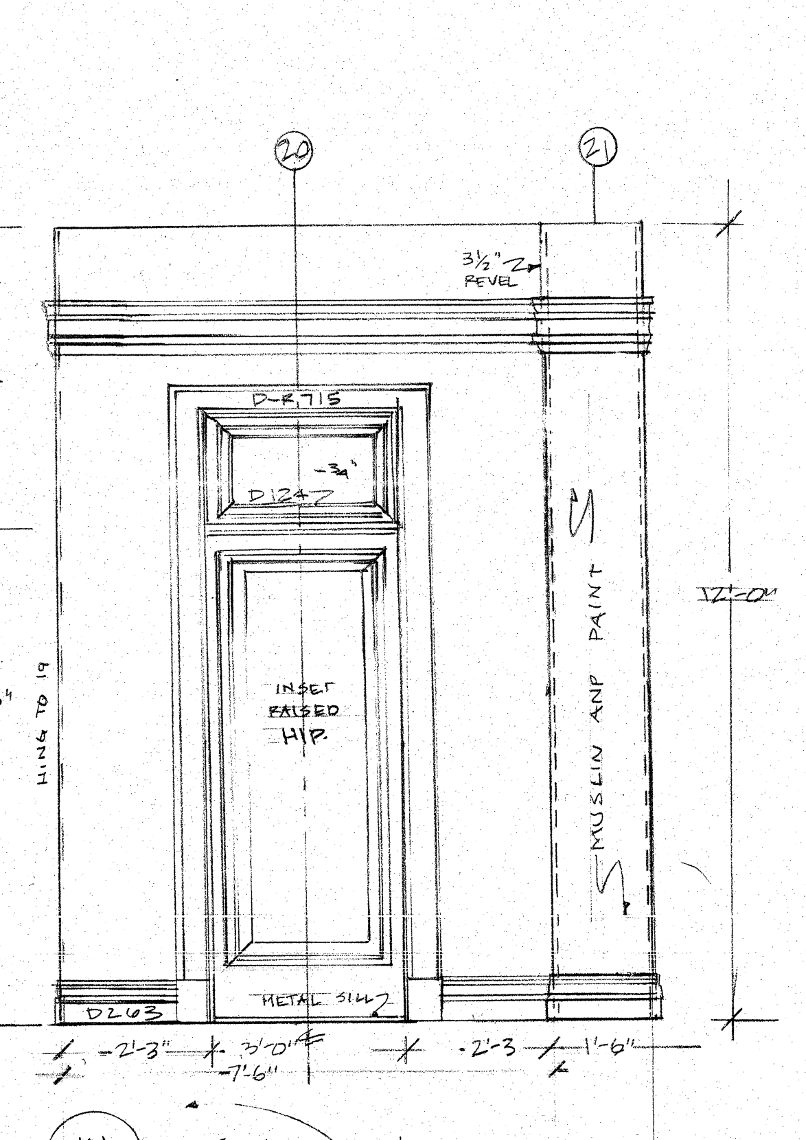
H. S. R. DOOR SCALE 1/2" = 1'-0"
