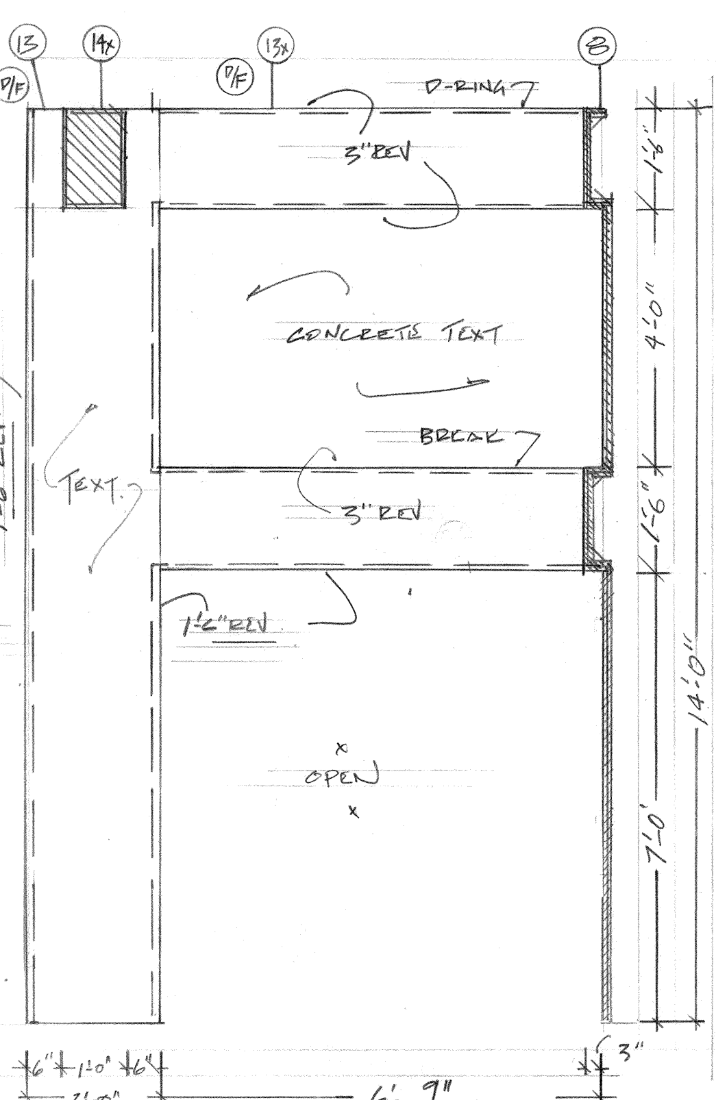
L D.S. COLUMN SCALE 1/2" = 1'-0"
