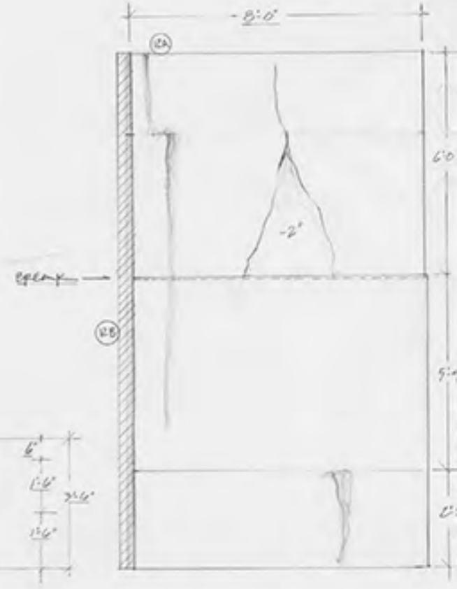
C DS LEFT WALL SCALE 1/8"=1'-0"
